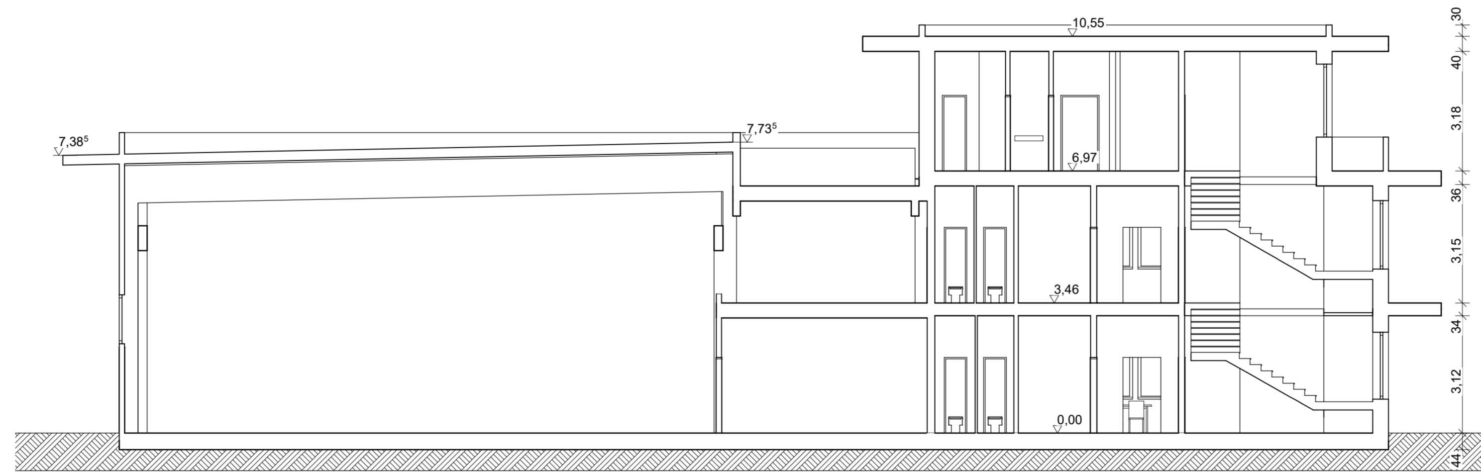
Schnitt B-B
