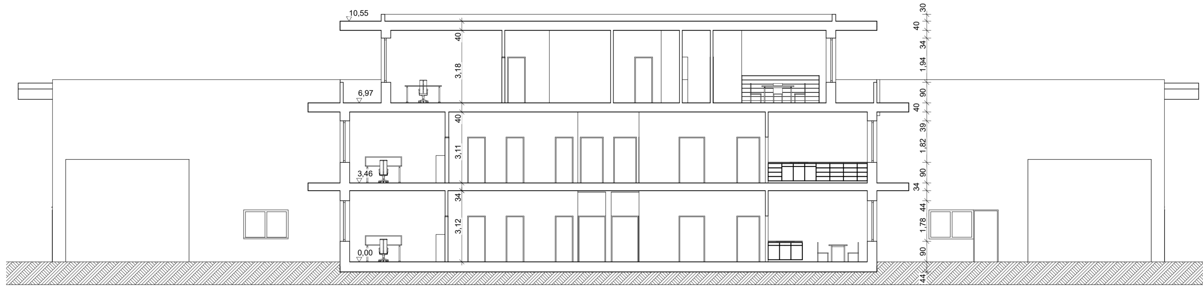
Schnitt A-A
